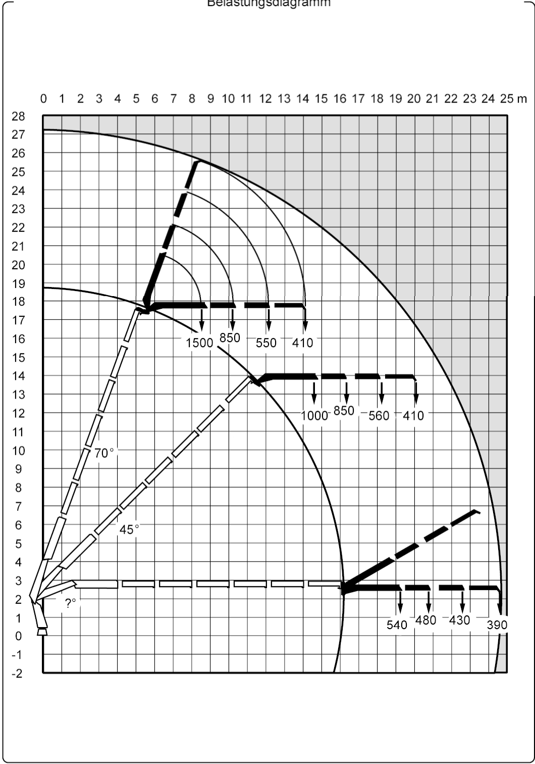
Belastungsdiagramm
