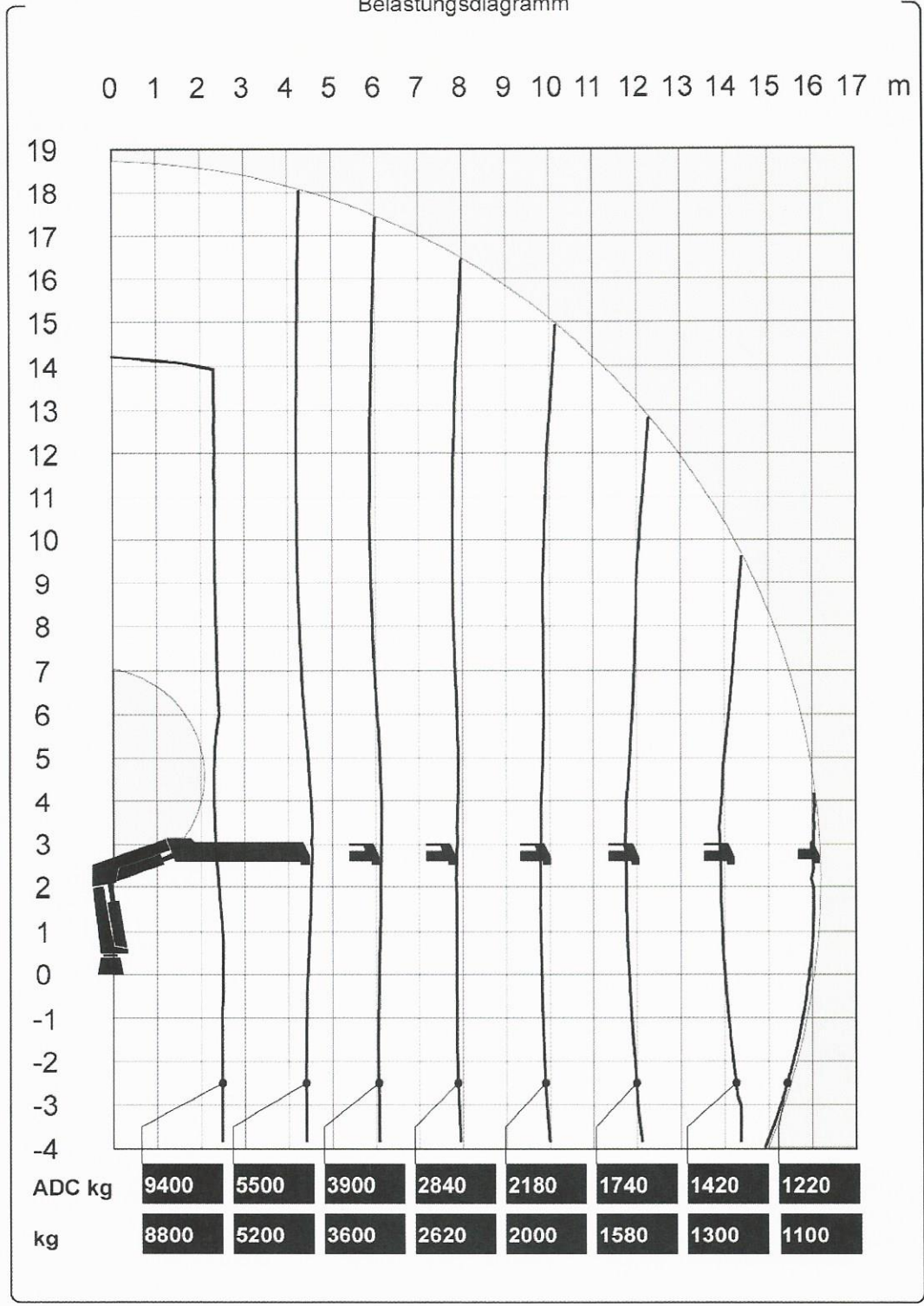
Belastungsdiagramm
